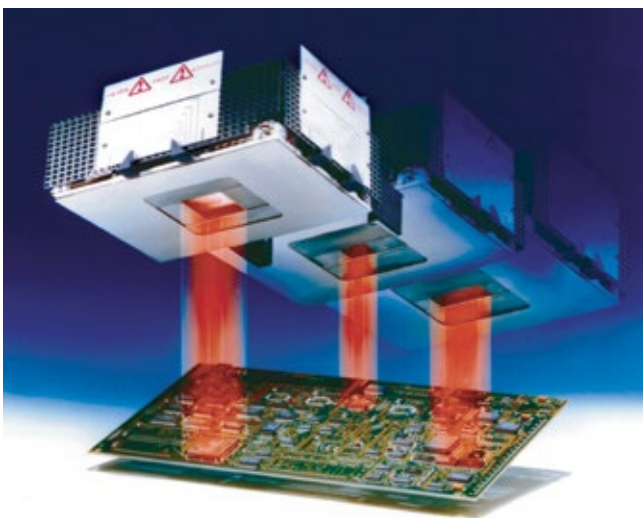
Bild 30: SMD-Lötkopf für Leiterplattenreparaturen
