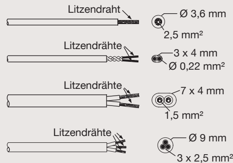
Elektro- und Temperaturregelungszubehör Einbaumaße und Abmessungen in mm
