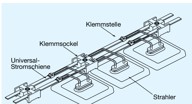
Bild 13: Schienenverdrahtung
