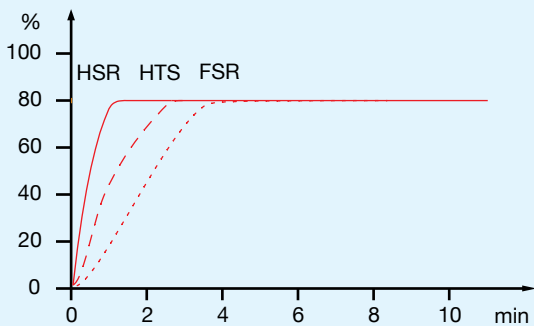
Bild 19: Leistung im geregelten Betrieb
